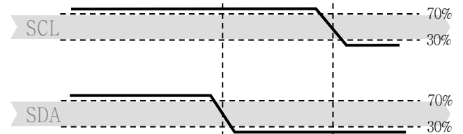
图 10 启动传输状态 (S) - 当 SCL 为高电平时，SDA 由高电平转换为低电平。开始状态是由主机控制的一种特殊的总线状态，指示从机传输开始 (Start 之后，BUS 总线一般被认为处于占线状态)
