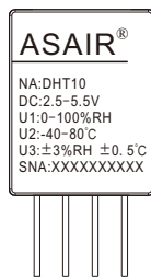
图 13 传感器激光标识。
